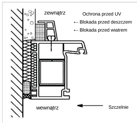
Rys. 27. Uszczelnienie dwustopniowe
