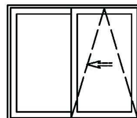
Okno / drzwi unoszono – przesuwno - uchylne
